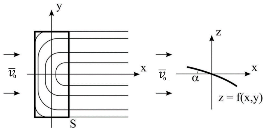
Рис. 1. Крыло в стационарном потоке невязкой несжимаемой жидкости
