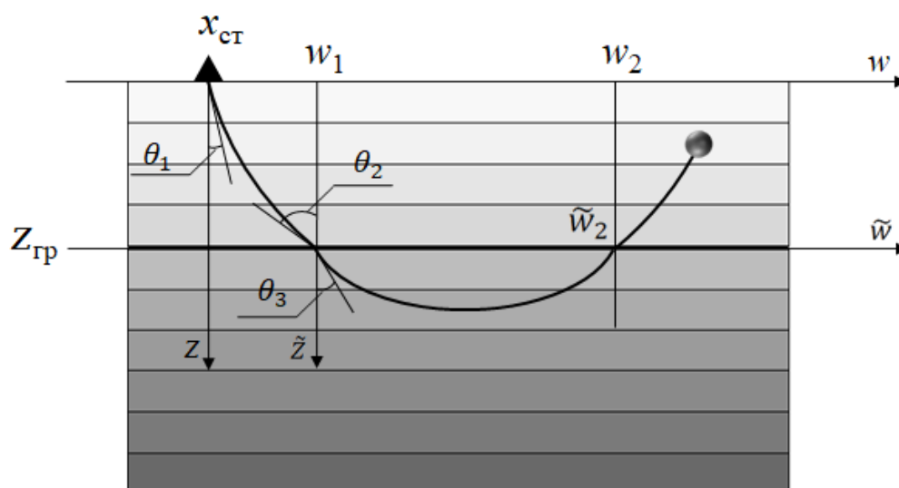
Рис. 1. Источник и приемник - окружность и треугольник, соответственно. Граница перехода луча из среды первого градиента в среду второго градиента указана горизонтальной прямой z_{\text{гр}} , \theta_1 – угол падения луча на приемник – сейсмическую станцию, \theta_2 – угол падения на глубину z_{\text{гр}} , границу между двумя градиентами, \theta_3 – угол преломления, определяющий распространение волны в среде второго градиента
