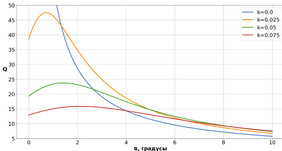
Рис.2. Зависимость аэродинамического качества от угла атаки
